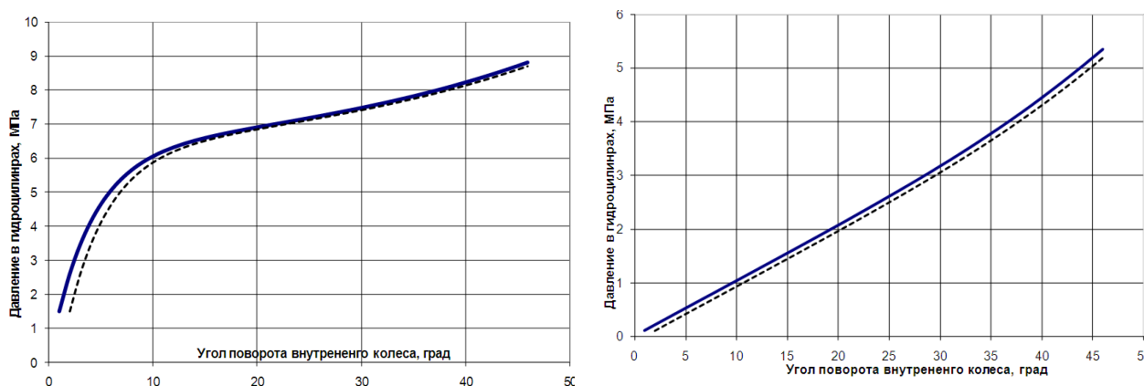
Рисунок 3 – Давление в гидроцилиндрах при повороте колес на месте и при круговом движении трактора в функции угла поворота внутреннего колеса
