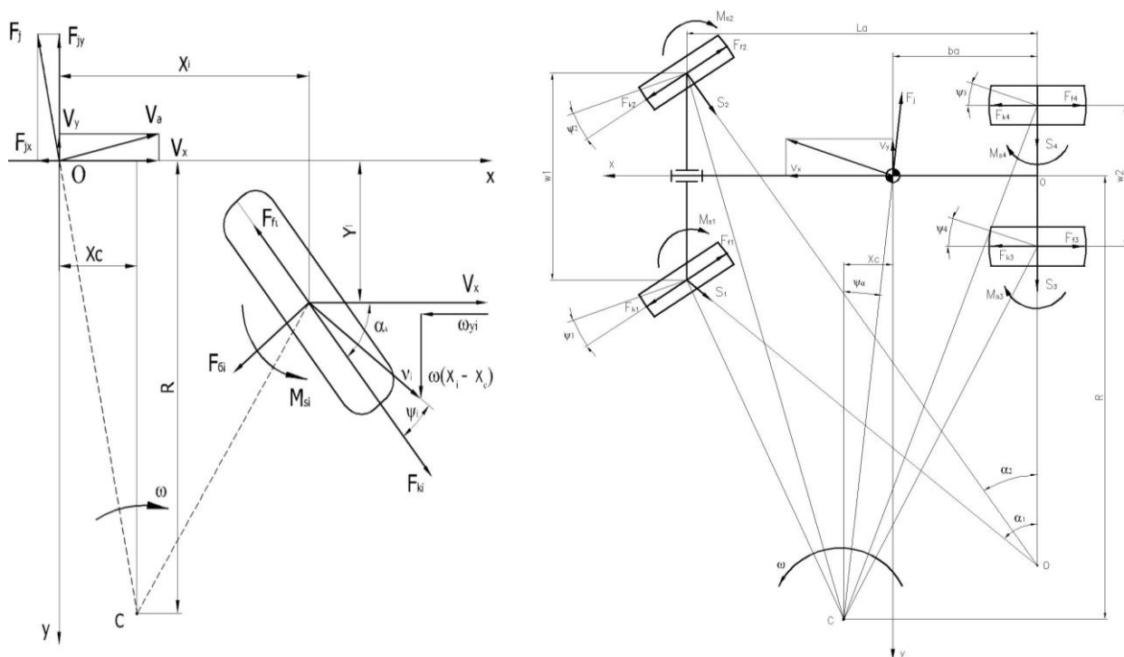
Рисунок 1 - Проекция колеса в плоскости дороги и схема сил, действующих на трактор
